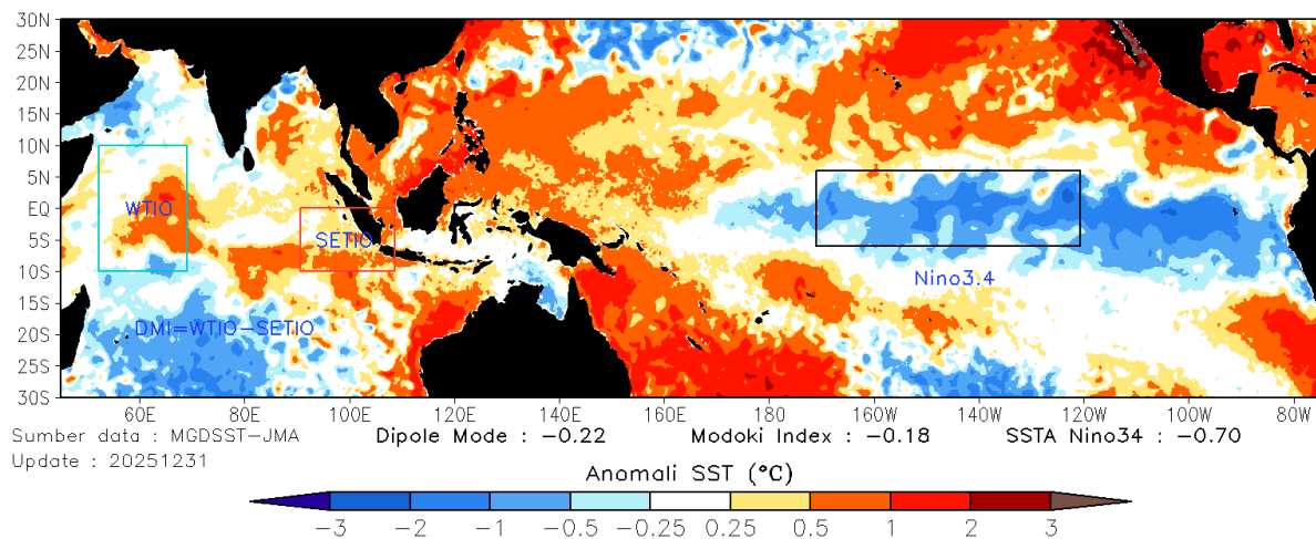
Gambar 3.2 Anomali Suhu Muka Laut di sekitar wilayah Indonesia pada Dasarian V bulan Desember 2025
